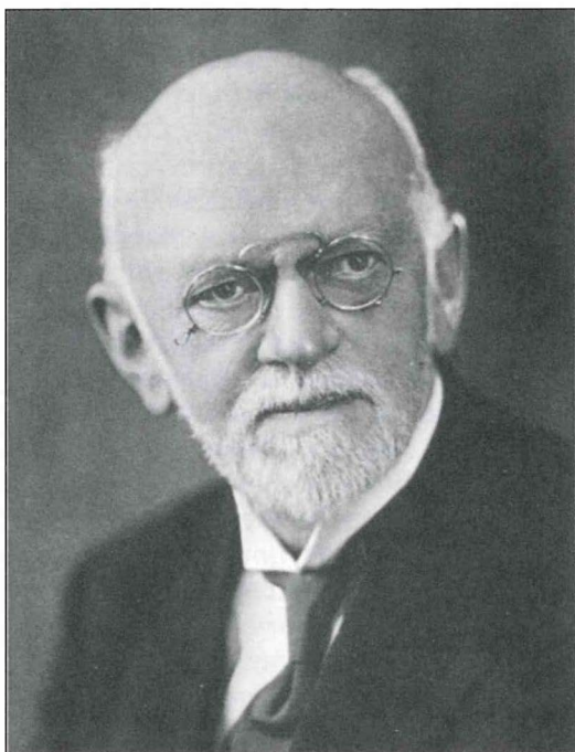
David Hilbert
